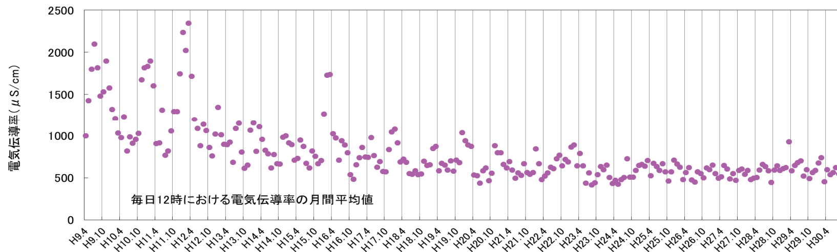
図-1 地下水No.2の電気伝導率の変化
