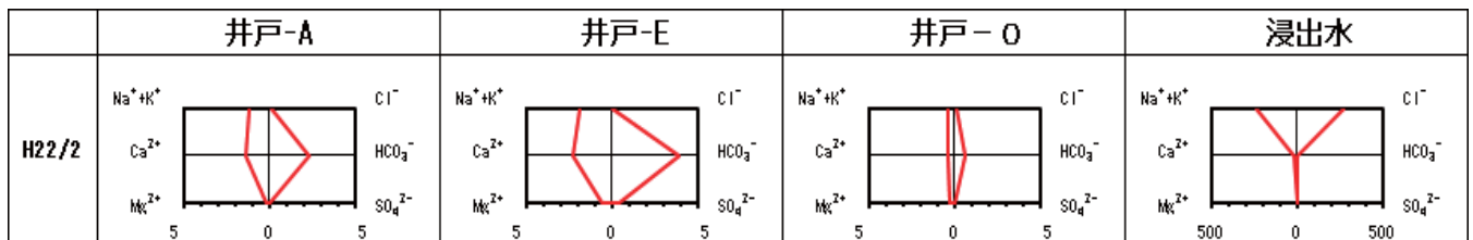
図-2 モニタリング井戸のイオンバランス（平成22年2月） 単位：meq/L
