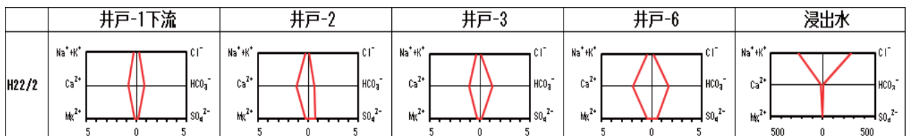
図-3 場外井戸のイオンバランス（平成22年2月） 単位：meq/L
