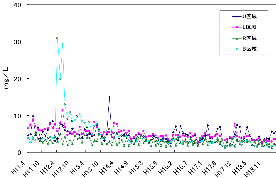
下流部観測孔各区域における塩化物イオン濃度(平均値)
