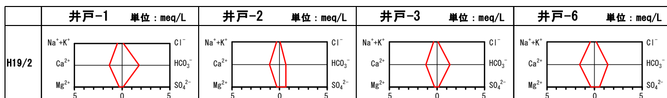
図-3 場外井戸のイオンバランス (平成19年2月)
