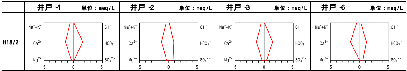
図 - 3 場外井戸のイオンバランス (平成18年 2月)
