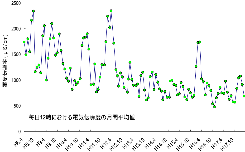
地下水管2水の電気伝導率の推移
