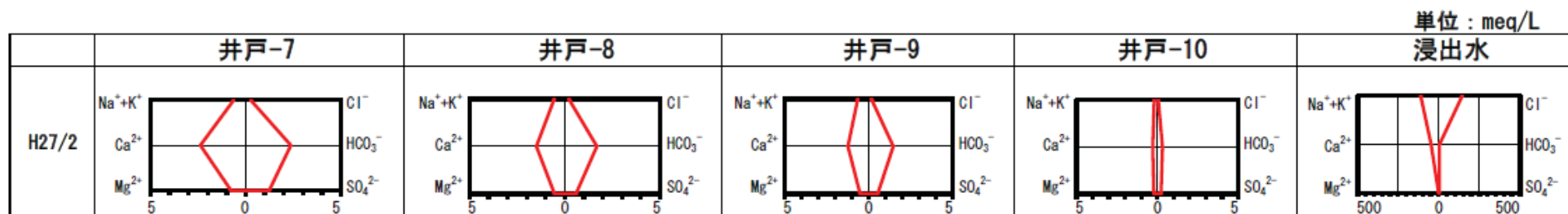
図-4 場外モニタリング井戸のイオンバランス
