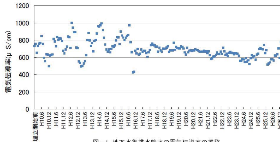
図一 地下水集排水管水の電気伝導率の推移
