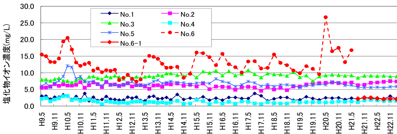
図-2 場内モニタリング井戸の塩化物イオン濃度の推移
