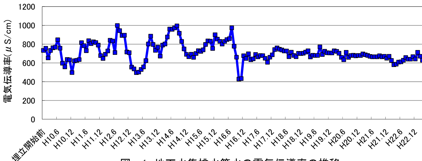
図-1 地下水集排水管水の電気伝導率の推移
